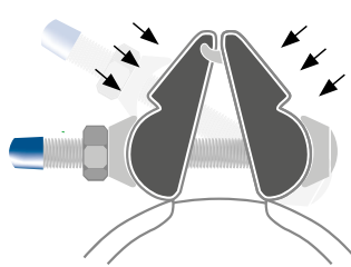
L'unique manchon de réparation équilibrant le refoulement du joint.
